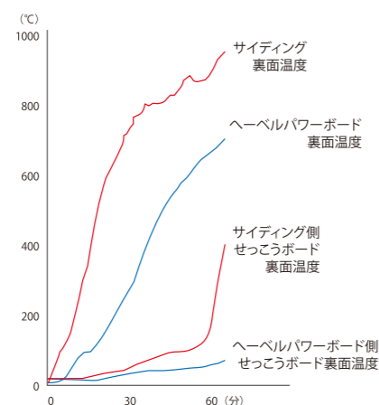
【外壁材裏面と内装せつこうボード裏面の温度変化】
